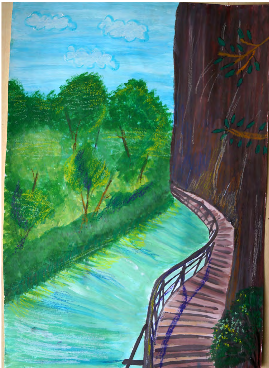
Река Златна Панега
